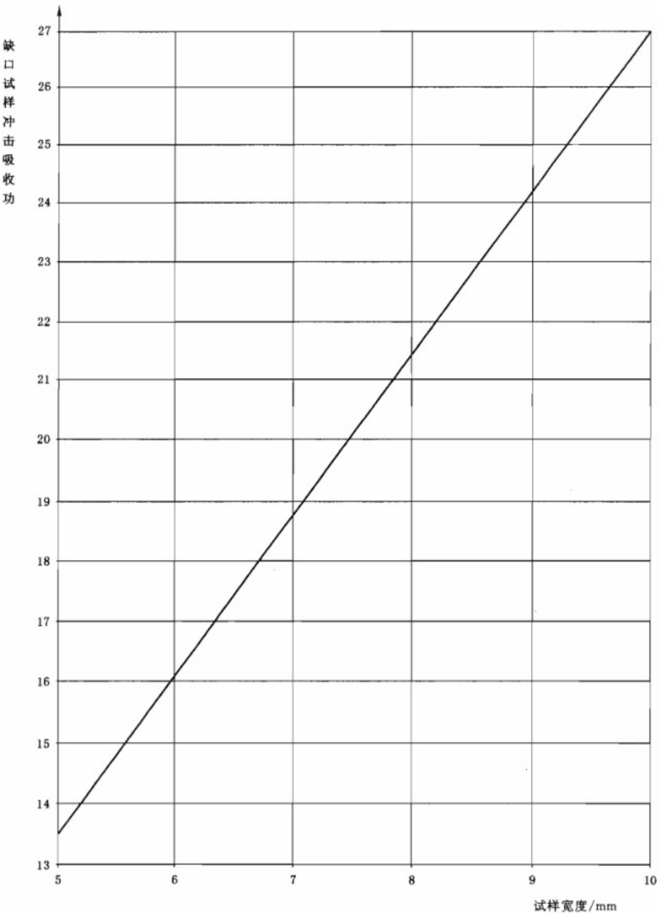
图 A.1 宽度 5 mm~10 mm 试样的最小冲击吸收功值
